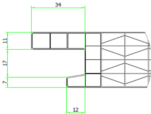
DETALLE LADO A ESCALA 1:1
