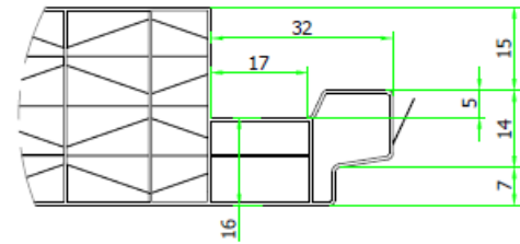
DETALLE LADO B ESCALA 1:1
