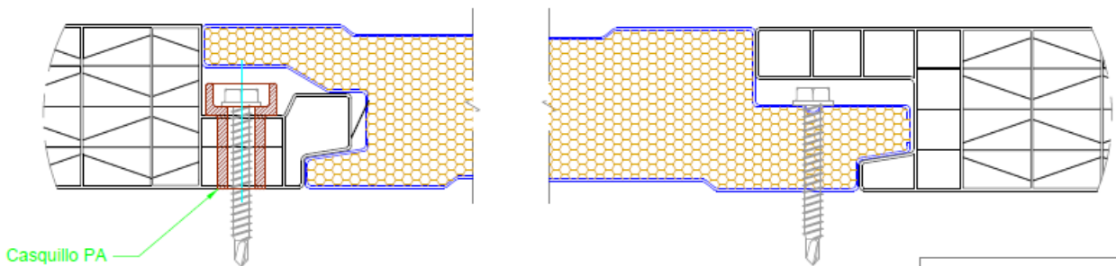
DETALLE ENCUENTRO CON METALPANEL FACHADA ESCALA 1:1
