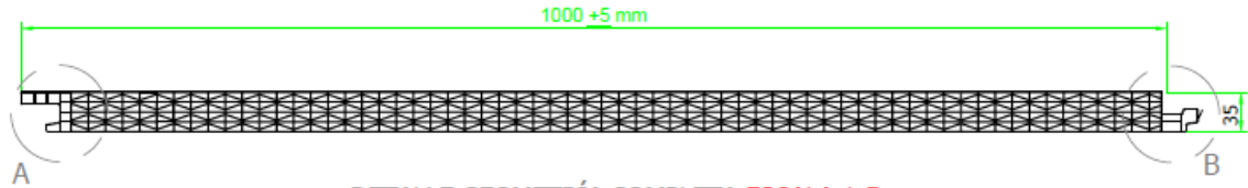
DETALLE GEOMETRÍA COMPLETA ESCALA 1:5
