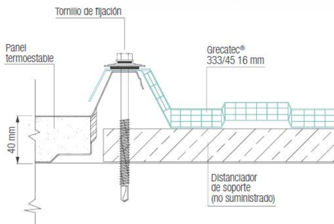
Detalle de fijación y solape lateral con Greca Tec® 333/45 16 mm
