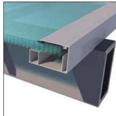
Detalle acabado lateral cubierta.
